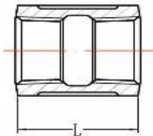
Рис. 2 - Муфта
